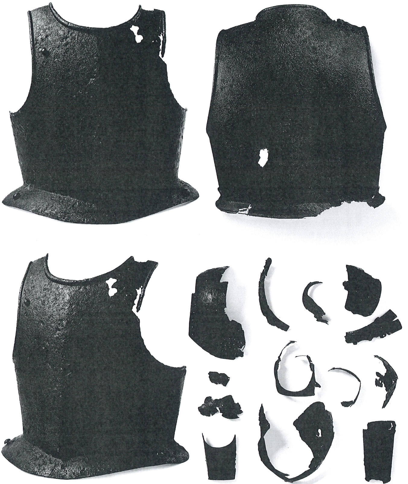
Fig. 2 Armour of Titore (Te Papa collection ME 001845).
